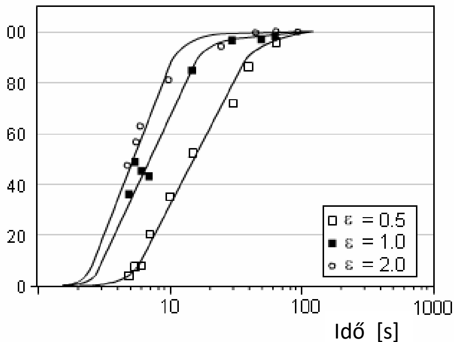
Rekrisztallizált hányad [%]
